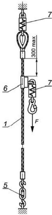
б — Пример испытаний жесткой анкерной линии, состоящей из проволочного каната
