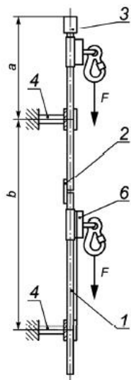
а — Пример испытаний жесткой анкерной линии, состоящей из рельса
